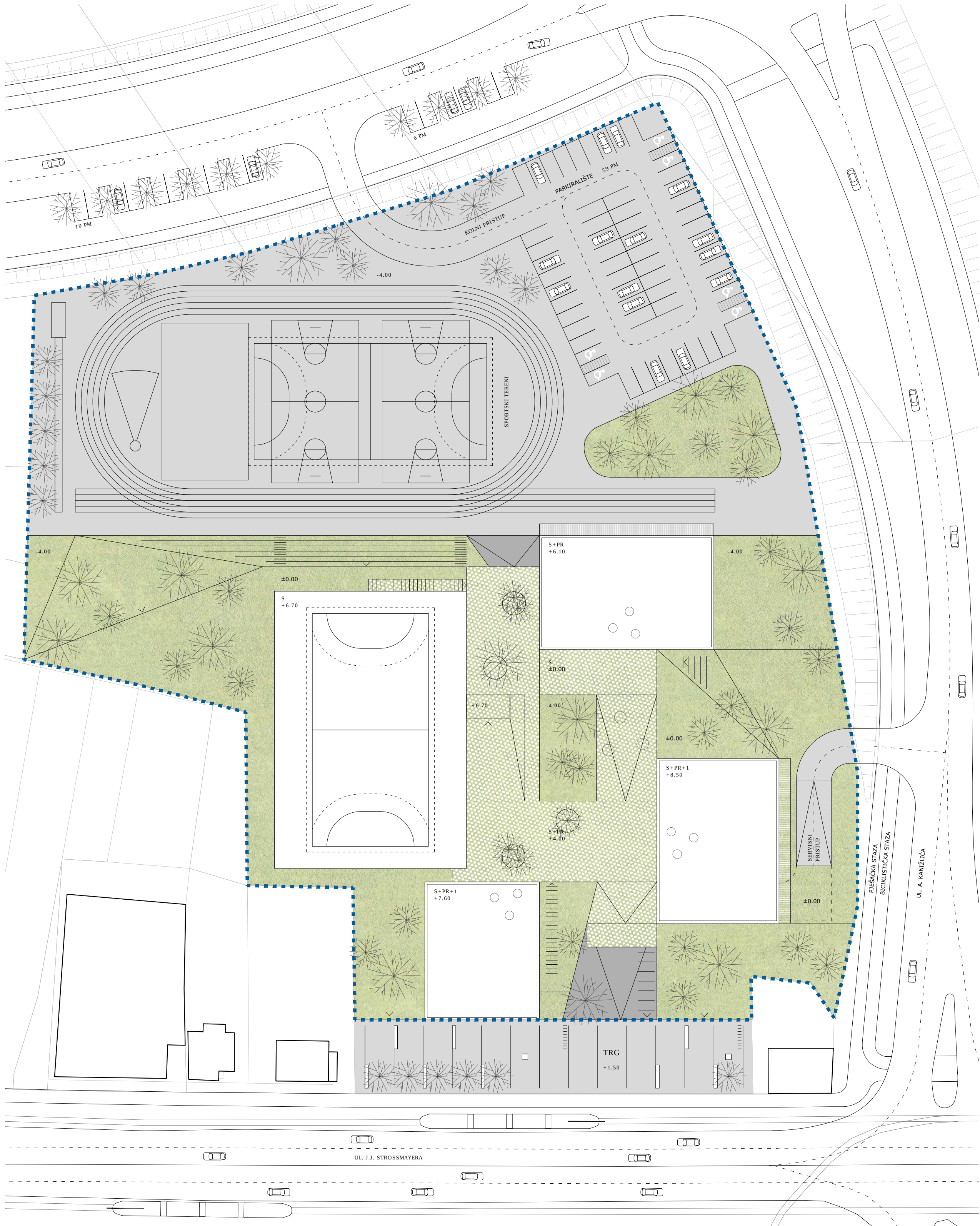
SITUACIJA S TLOCRTOM KROVA MJ 1 | 500
