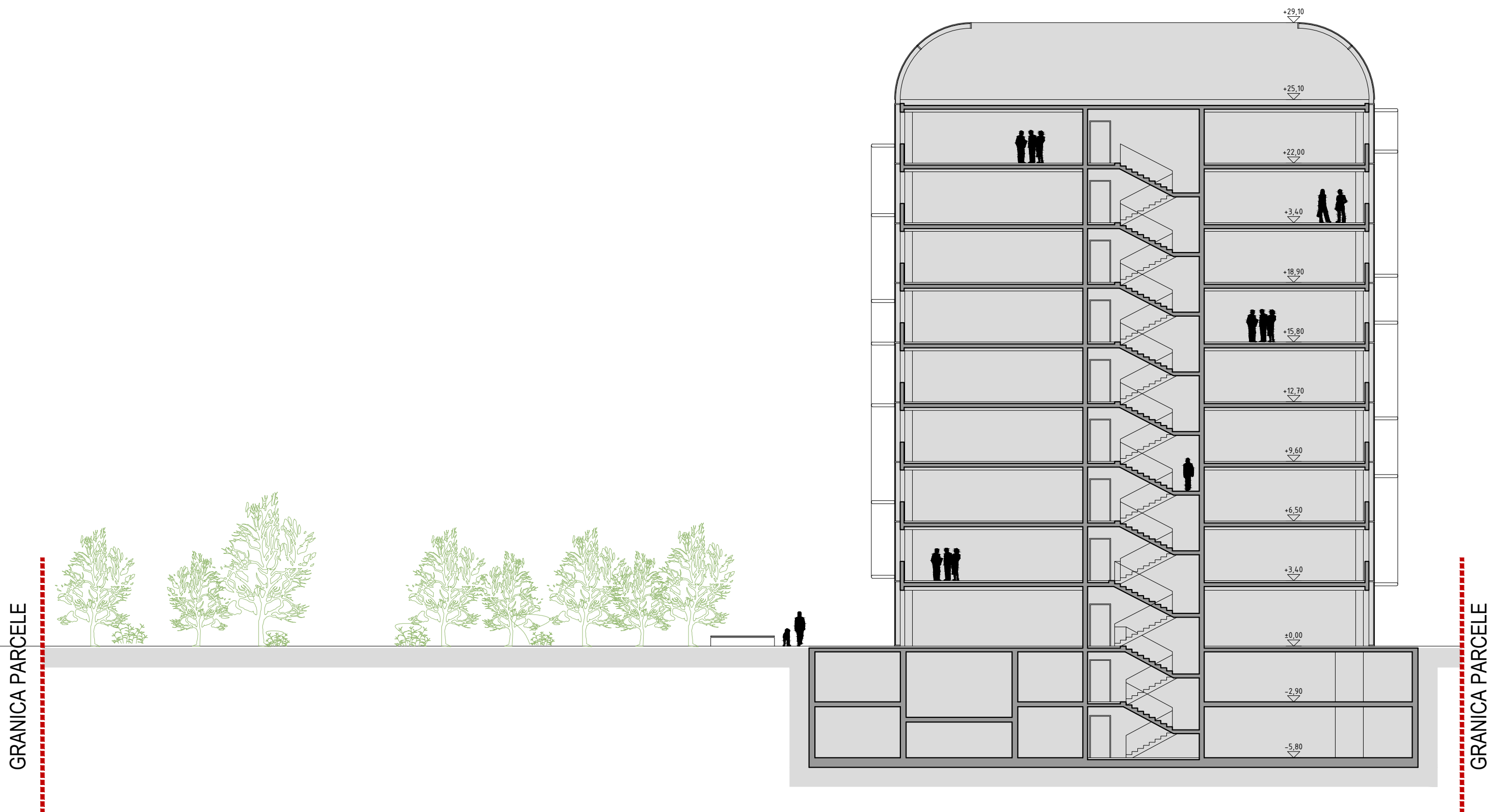
PRESJEK C-C
