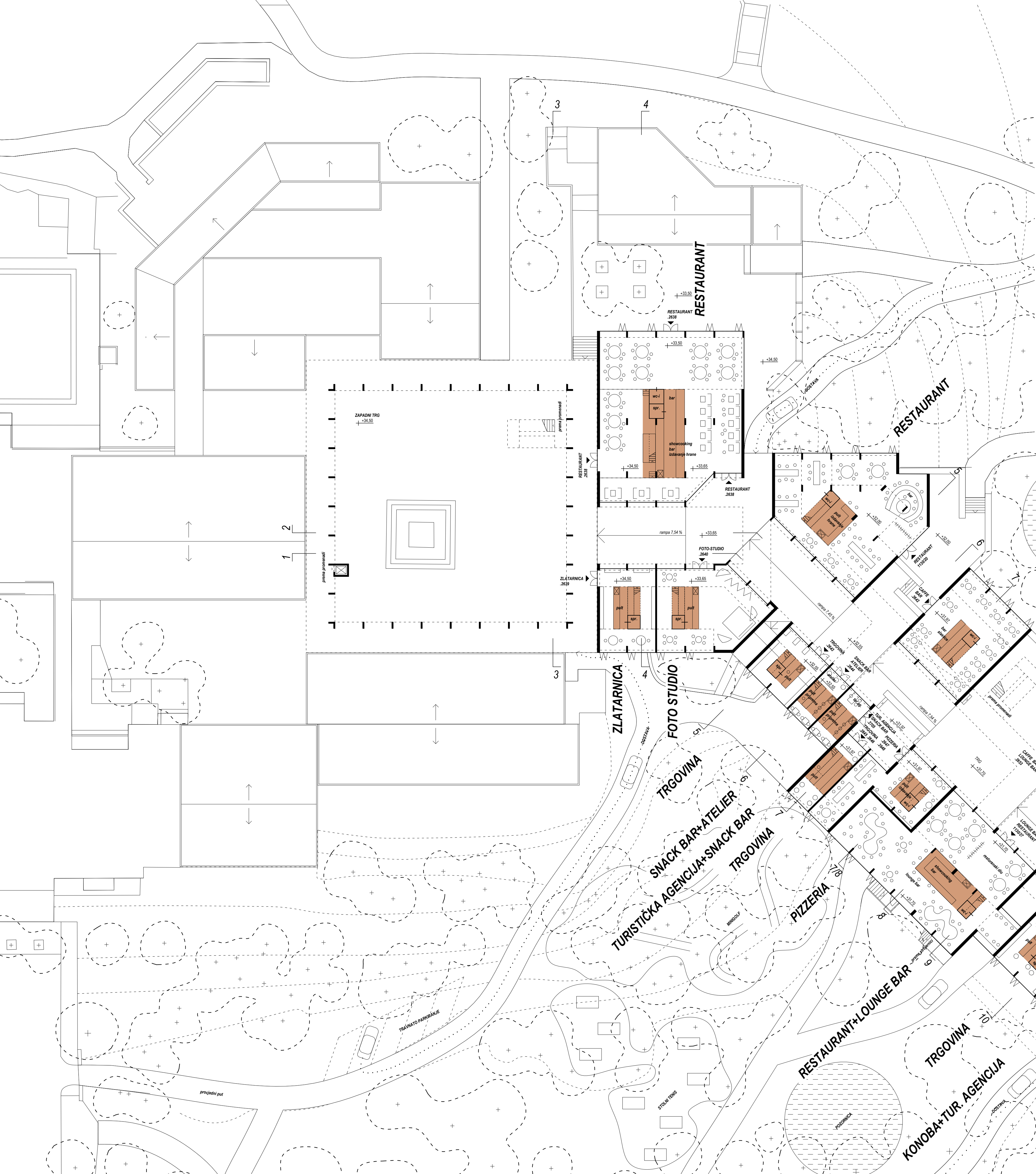
SITUACIJA S TLOCRTOM PRIZEMLJA i naznačenim prostorno-funkcionalnim cjelinama M1:250 > oslobođeno prizemlje s jezgrama
