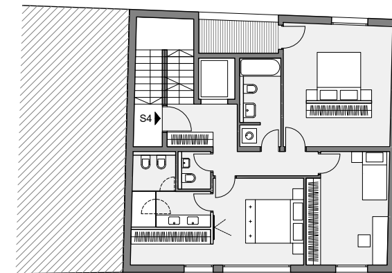
TLOCRT 4. KATA
