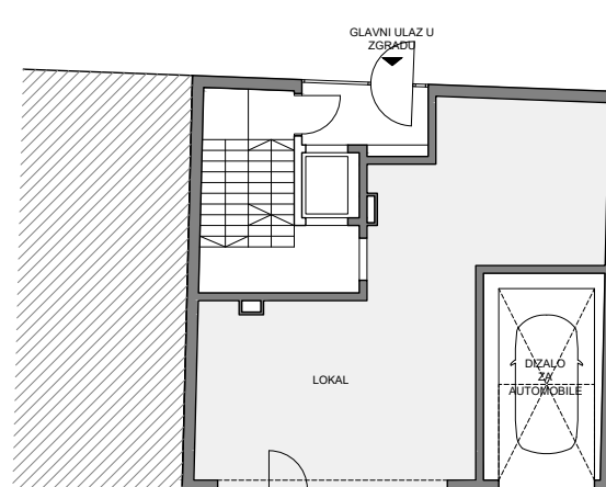
TLOCRT PRIZEMLJA
