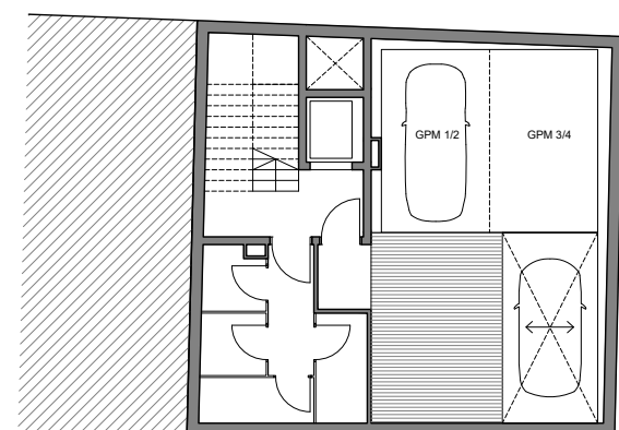
TLOCRT PODRUMA
