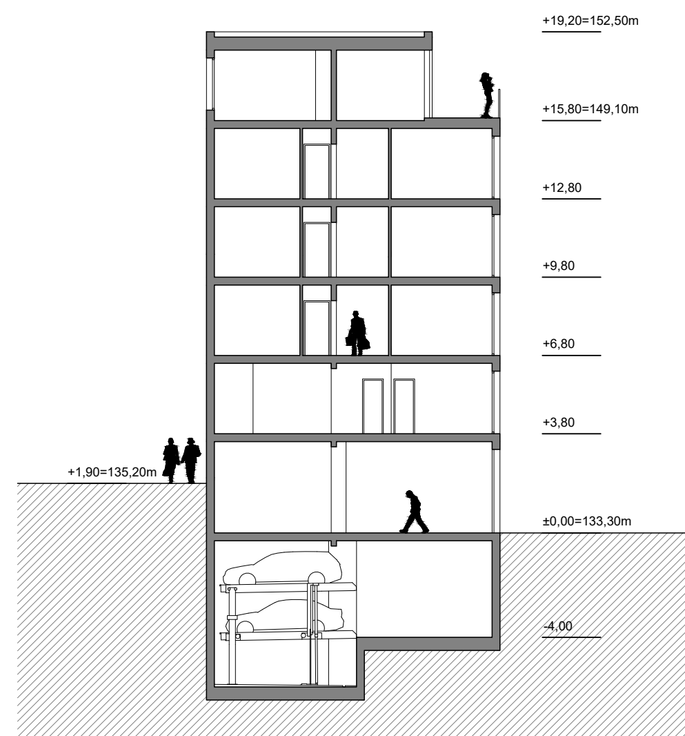
PRESJEK A-A
