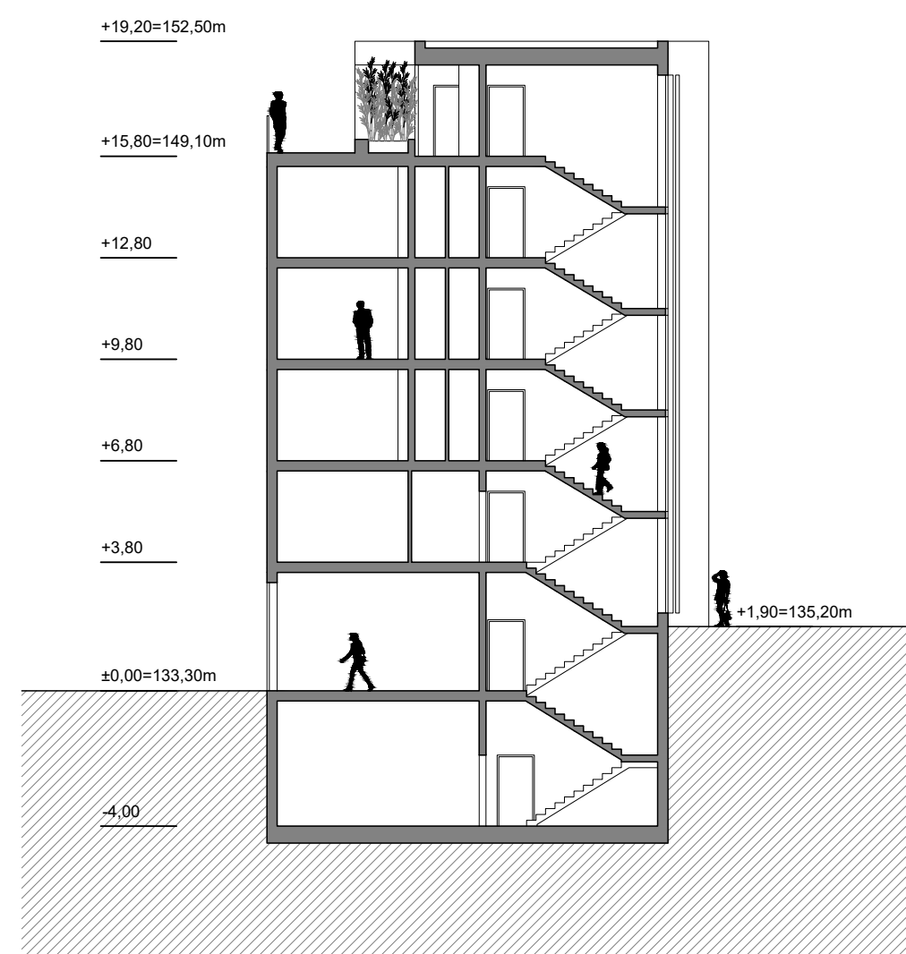
PRESJEK B-B
