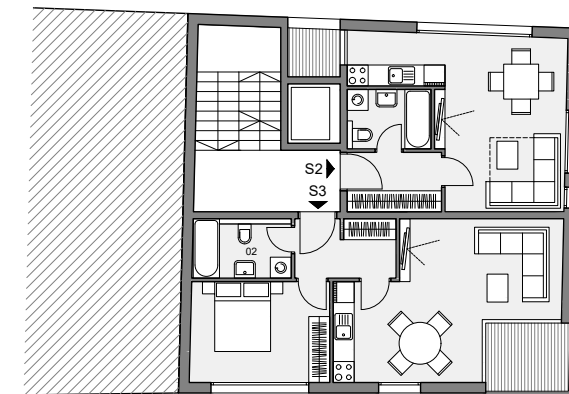
TLOCRT 3. KATA
