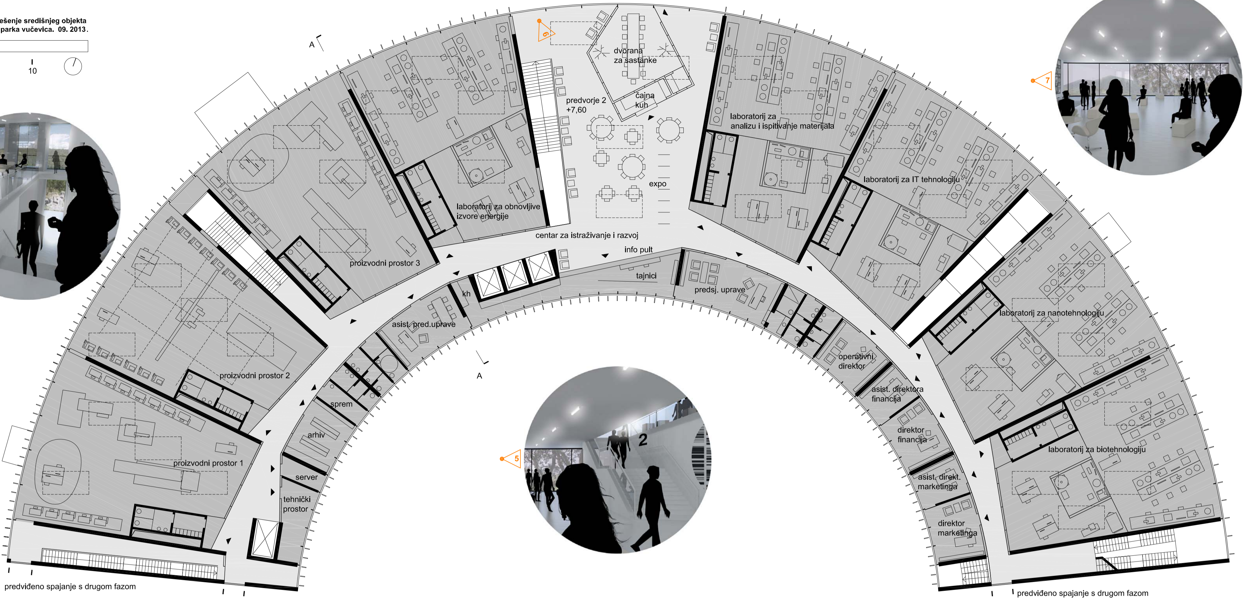
tlocrt 2. kata
