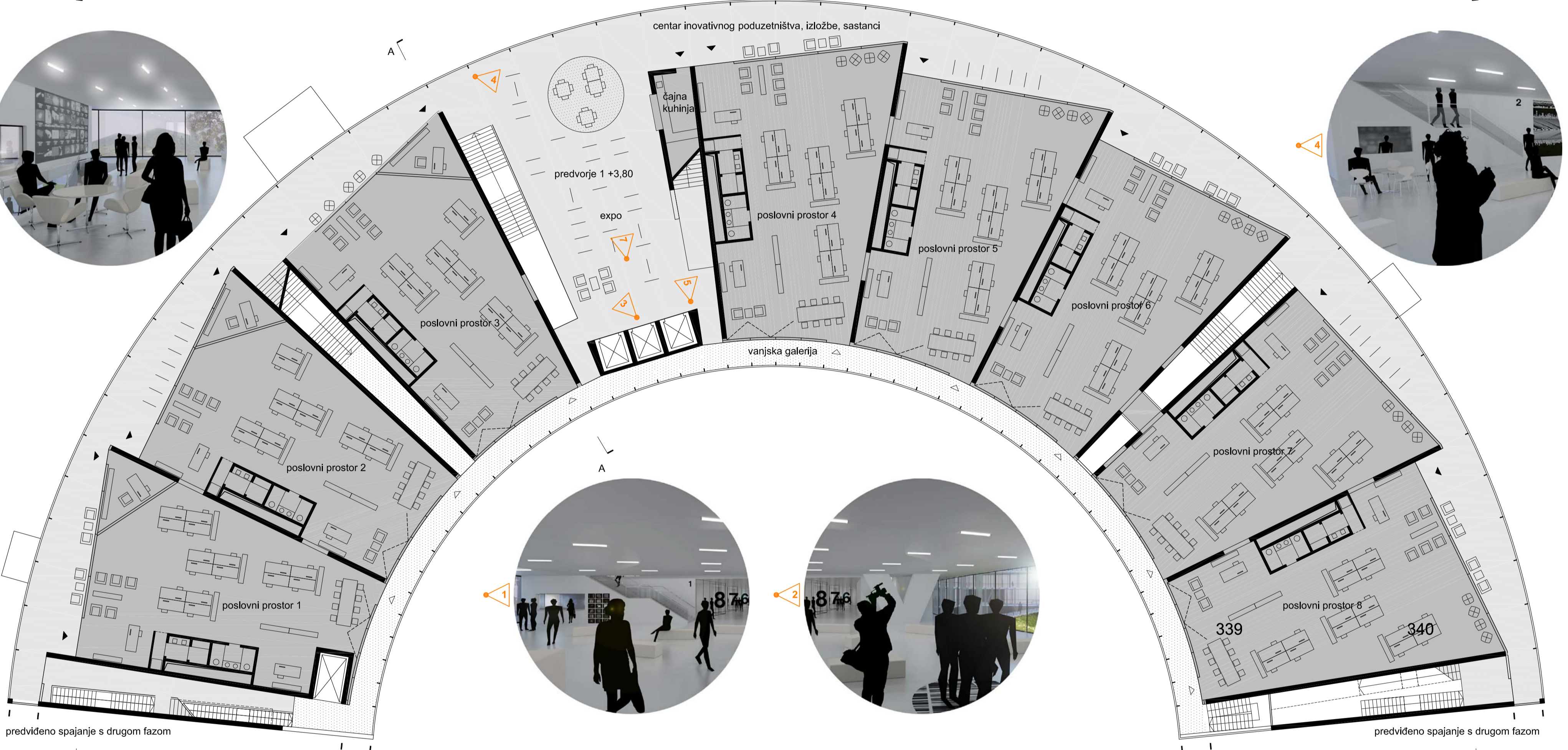
tlocrt 1. kata
