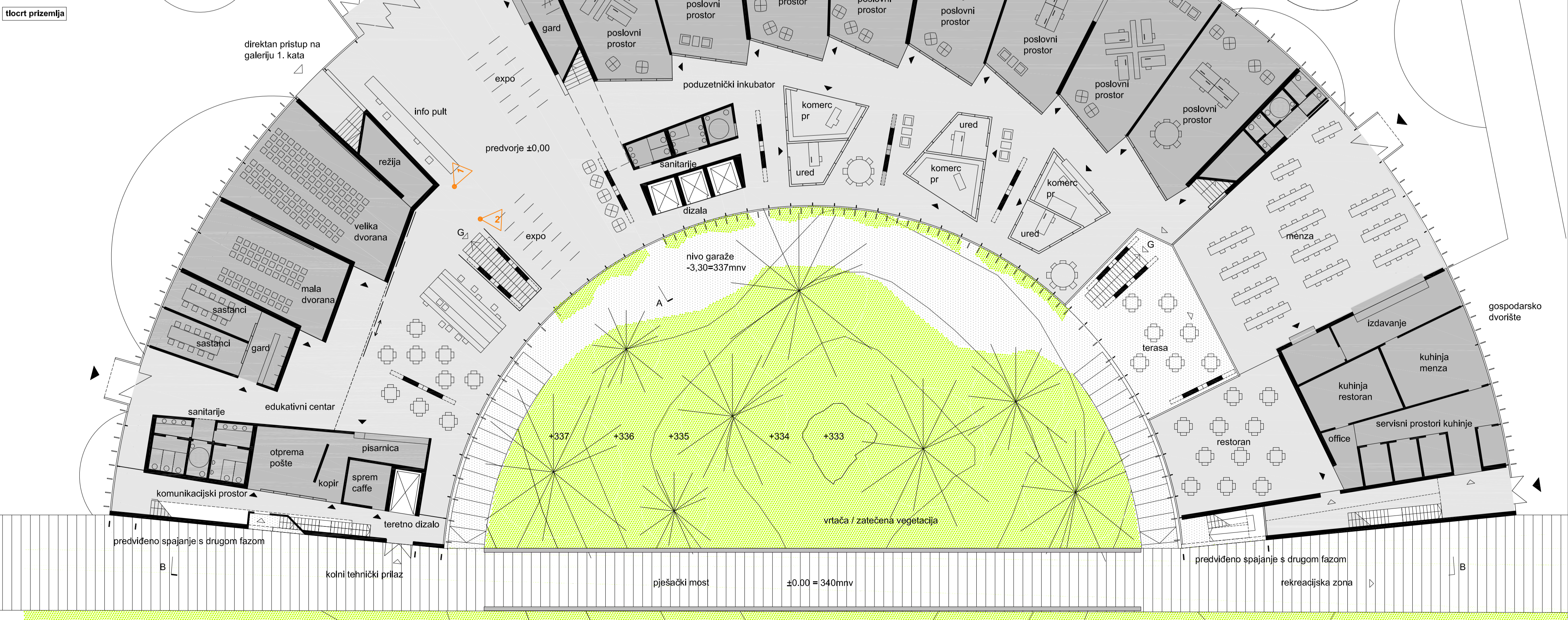
tlocrt prizemlja
